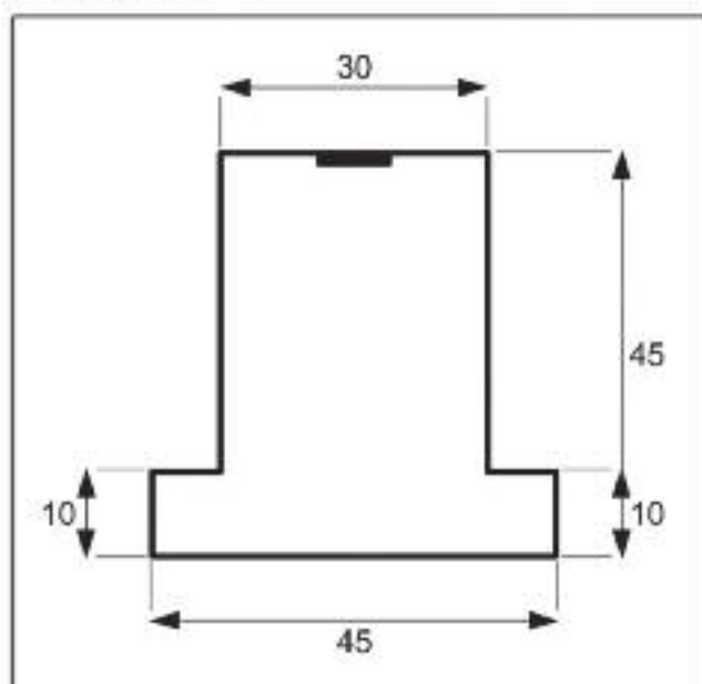
Sezione profilo
